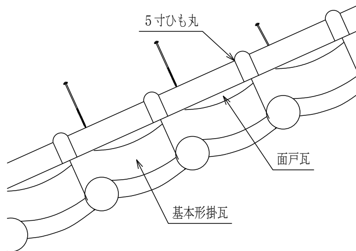
掛け瓦詳細図
